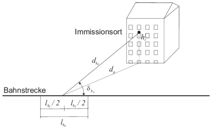
Bild 2: Definition des Winkels \delta_{k_s} an einer Bahnstrecke
