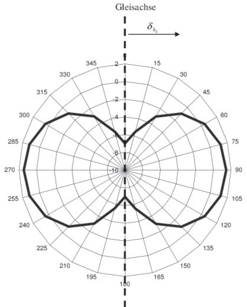
Bild 3: Richtwirkungsmaß D_{I,k_s} in dB nach Gleichung (Gl. 8) für \delta_{k_s} in Grad
