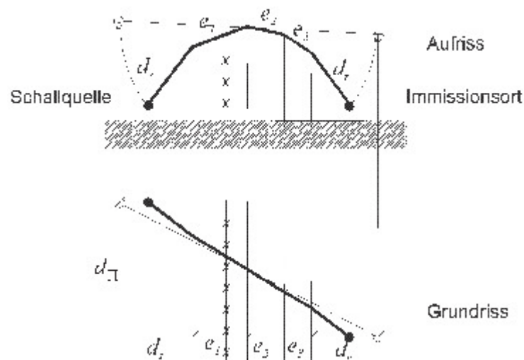
Bild 6: Beispiel für einen Schallweg über mehr als zwei maßgebliche parallele Beugungskanten; zu vernachlässigende Kanten sind durch x markiert. Die Auswahl der maßgeblichen Beugungskanten erfolgt nach der sogenannten Gummibandmethode. Kanten, die von einem Gummiband, das von der Punktschallquelle zum Immissionsort gespannt wird, nicht berührt werden, bleiben für die Mehrfachbeugung unberücksichtigt. Bei nicht parallelen Beugungskanten, d. h. wenn mindestens eine Beugungskante nicht parallel zu den übrigen am Gummiband beteiligten Beugungskanten ist, gilt:
