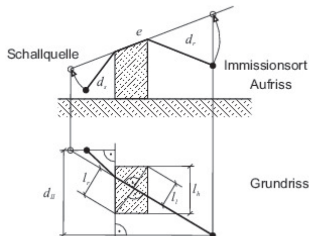
Bild 5: Schallweg über ein Hindernis mit zwei wirksamen parallelen Kanten Eine Schirmkante, über die der Schall hinweg gebeugt wird, ist dann als Oberkante zu bezeichnen, wenn sie mit der Horizontalen einen Winkel von weniger als 45^\circ
